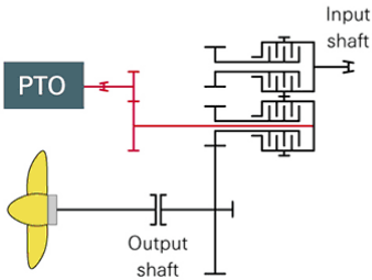
Top PTO72 (R*+NR*Version)
