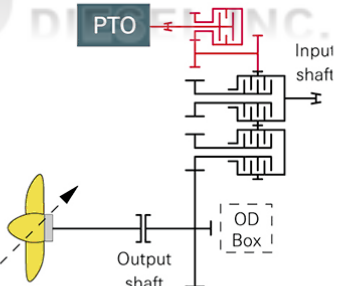
Top PTO74 (R*+NR*Version)
