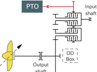
Top PTO74 (R*+NR*Version)
